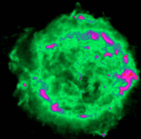
Radio (VLA)
