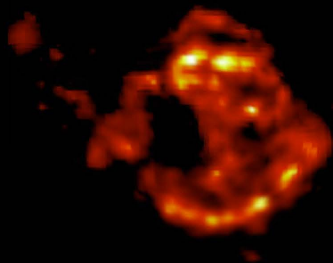
Infrared (ESA/ISO, CAM, P. Lagage et al.)
